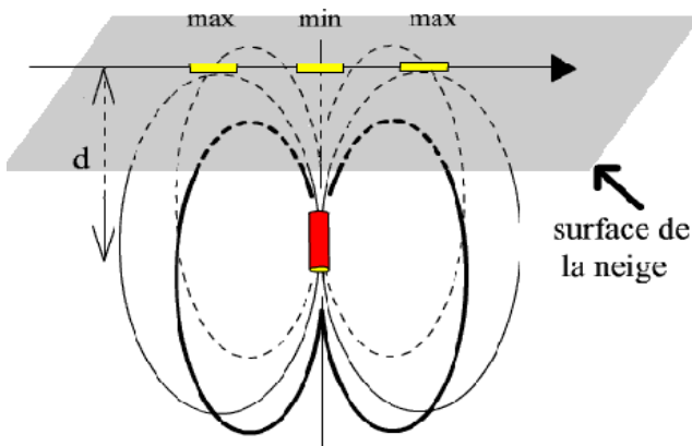
figure 5: Lignes de champ en 3D pour un DVA enfoui en position verticale, assez rare. Si on se déplace en ligne droite sans tourner le DVA, on enregistre deux maxima. Le DVA enfoui se trouve entre deux maxima.
