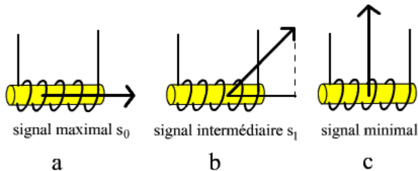
figure 2: Variation du signal en fonction de l'orientation du récepteur. a : Le champ est parallèle à l'antenne, le signal est maximum. b : Le champ est à 45°, le champ « vu par le détecteur » est divisé par \sqrt{2} = 1,414 . c : Le champ est perpendiculaire, le signal est nul.
