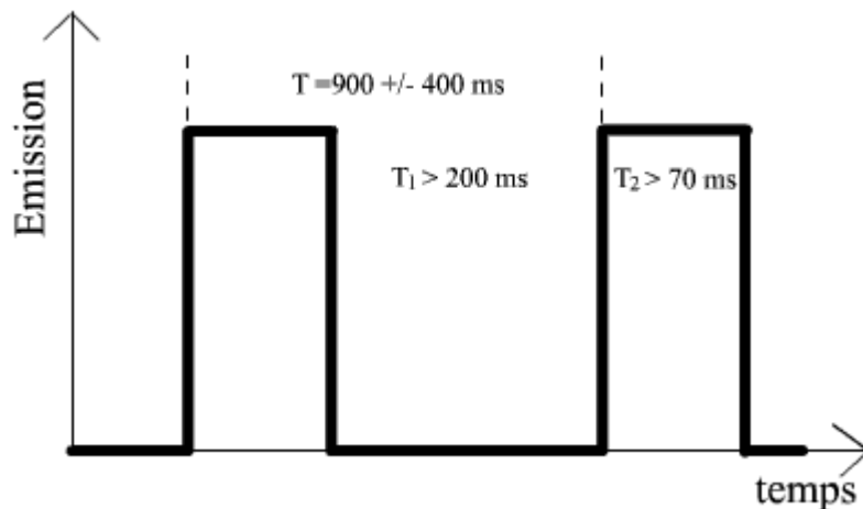
figure 1: Structure périodique de l'émission d'un DVA. Les durées T1, T2 et T peuvent varier d'un appareil à l'autre, les limites indiquées sont celles de la norme européenne ETS 300718.
